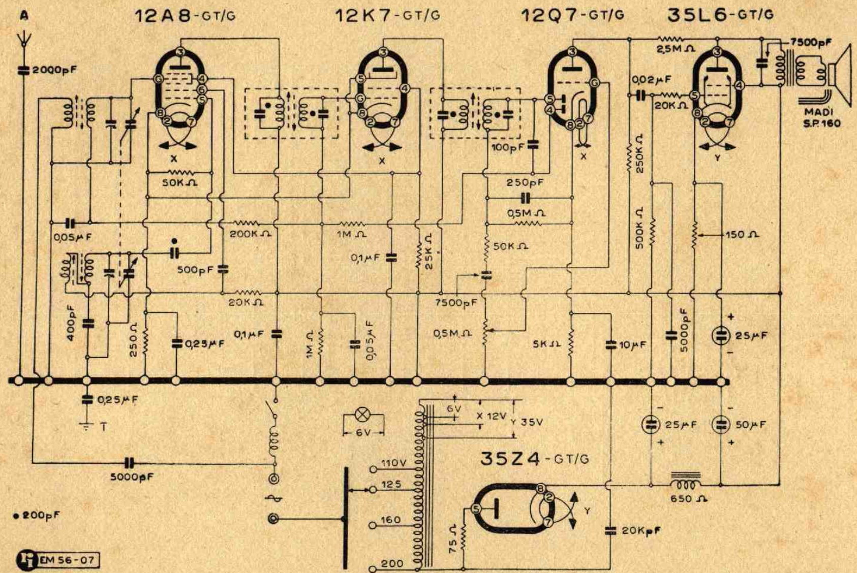
Lo schema elettrico del mod. AR 48
